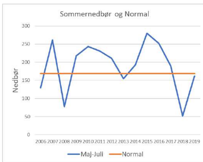
Figur 2b: Middelsommernedbør og normal for maj-juli.
