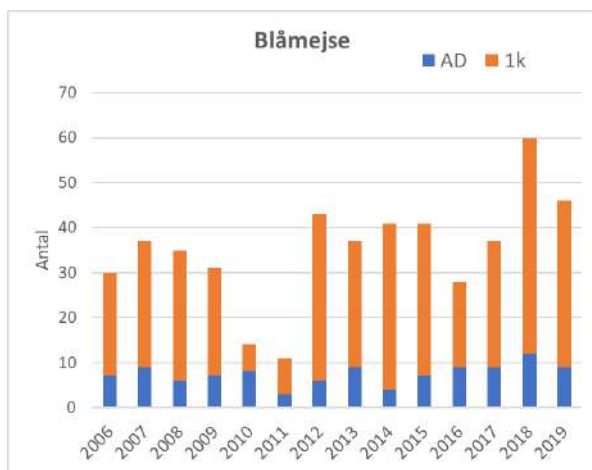
Figur 7. Antal blåmejsen fanget fordelt på år og alder.
