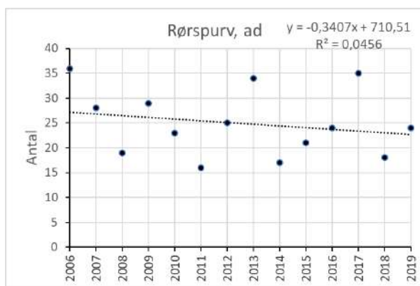
Figur 18 a. Antal adulte rørsurve fanget i perioden 2006-2019 (trendlinie indtegnet).
