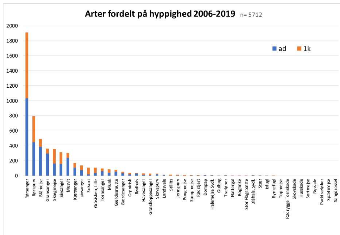
Figur 4. Fordelingen af de ringmærkede og aflæste 46 arter fanget i perioden 2006-2019 fordelt på fangsthyppighed.
