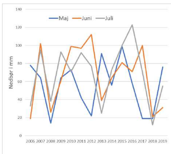
Figur 2a: Månedsmiddel nedbør for månederne maj-juli.
